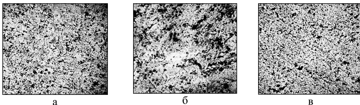
Рисунок 9 – Мікроструктури ( \times 400 ) зразків зі сплаву АК5М2, відлитих в НТФ при -20\text{ }^{\circ}\text{C} (а), в ПГФ при +20\text{ }^{\circ}\text{C} (б), в кокіль при +120\text{ }^{\circ}\text{C} (в)
